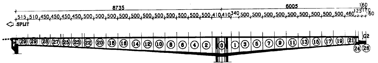
Slika 15. Izvedba prednapetog sklopa u odsječcima
