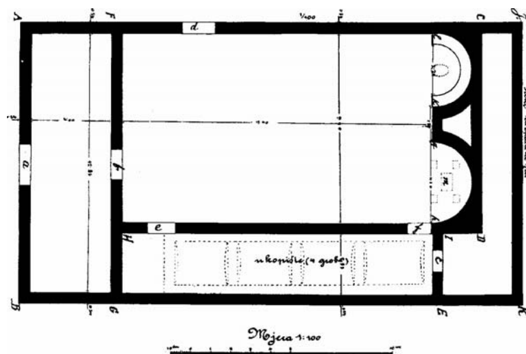
Stari tlocrt Crkvine u Bublínu u Zmijavcima (J. Mihulka)
