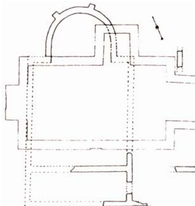
Suvremeni tlocrt stare crkve na groblju u Muću Gornjem (prema Marasoviću)
