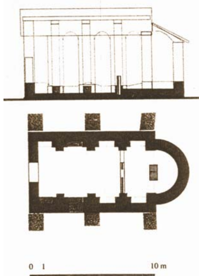
Presjek i tlocrt rekonstrukcije crkve Sv. Ivana u Uzdoľju
