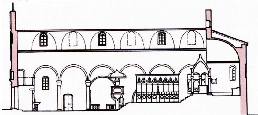
Presjek crkve Sv. Marije Velike
