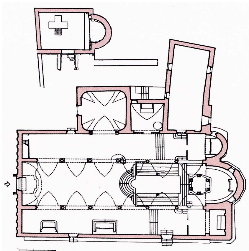
Tlocrt sadašnje nadžupne crkve Sv. Marije Velike. Naznačene su konture starokršćanske crkve, a krstionica je gore lijevo
