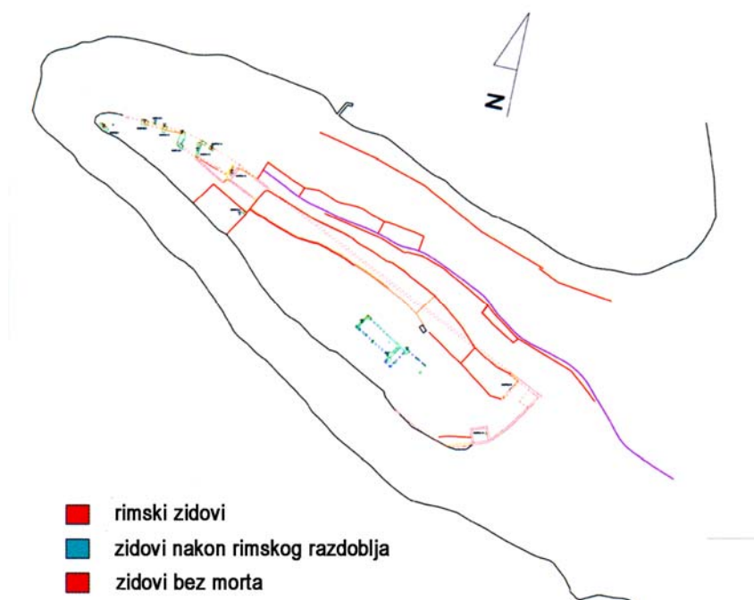
Tlocrt sadašnjih istraživanja ruševina na Kaštelini
