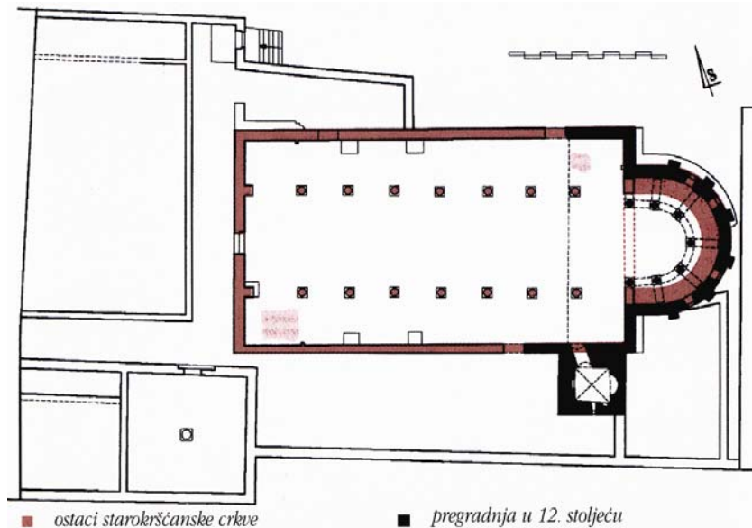
Tlocrt ostatka crkve i samostana Sv. Ivana Evanđelista
