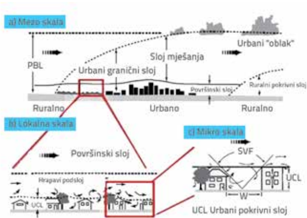
Slika 2. Termalni slojevi [19]
