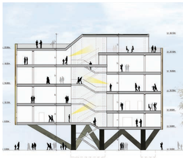
Presjek zgrade Humboldt Box
