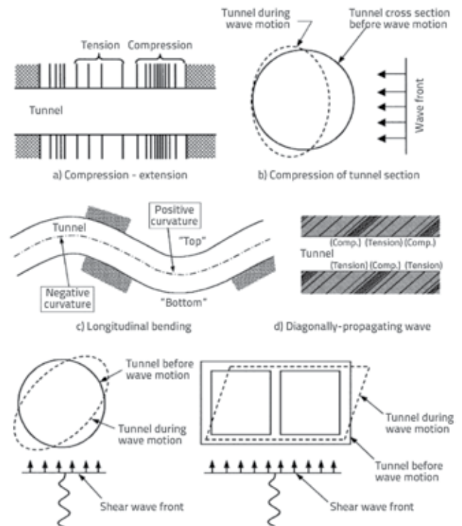
Slika 8. Primjeri deformacije tunela uslijed potresnog djelovanja [18]
