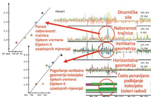
Slika 6. Korespondirajuće progresije naboranosti tračnica i vertikalne geometrije kolosijeka u vremenu i višestruko (nepotrebno) ponavljano podbijanje kolosijeka
