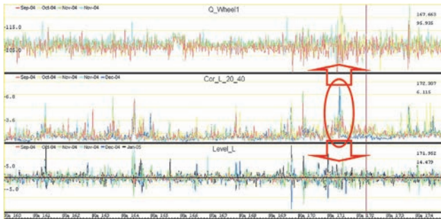
Slika 5. Posljedice naboranosti tračnica
