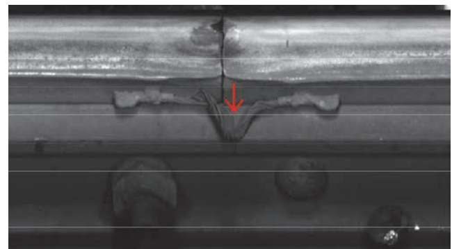
Slika 14. Nadzor tračnice i njenih komponenti – napuknuće veze [11]
