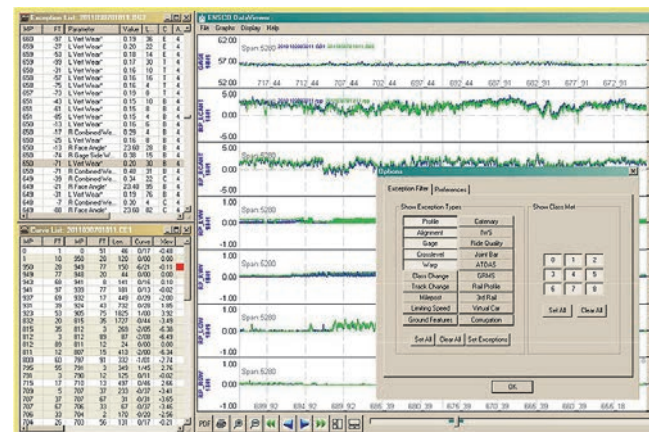
Slika 2. Primjer "sirovih" mjernih podataka za geometriju kolosijeka
