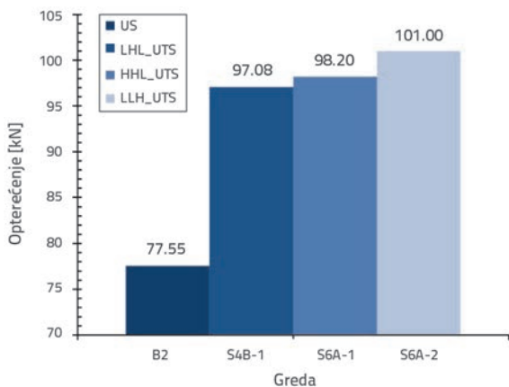
Slika 9. Granična nosivost običnih i ojačanih nosača bez obrađivanja površine
