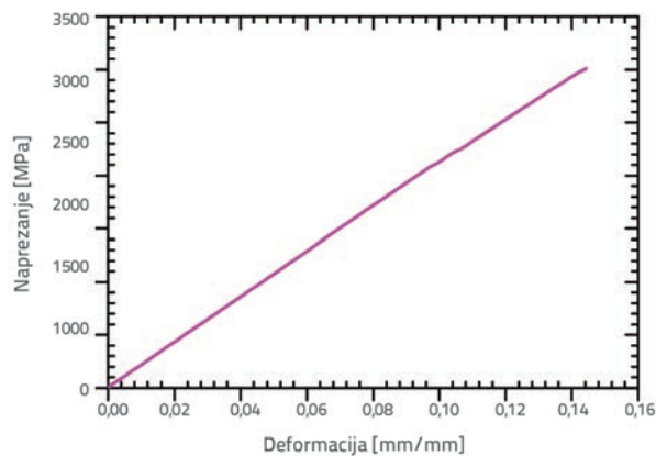
Slika 4. Dijagram naprežanje-deformacija za CFRP
